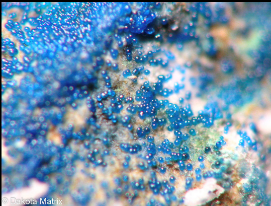
Santarosasite - Chile
